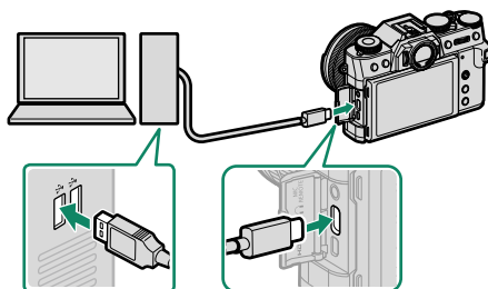
USB 连接插孔 (C 型)
