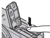
배터리 고정레버
