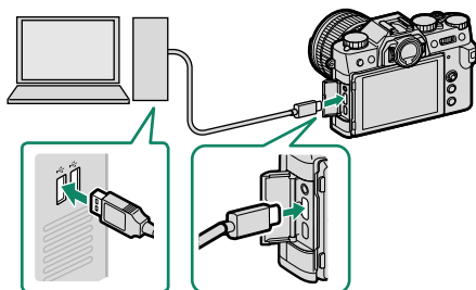
USB-Anschluss (Typ-C)
