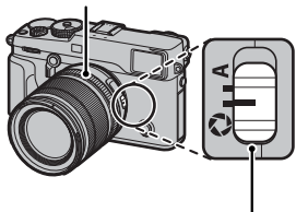
Diafragmastandenschakelaar
