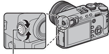
Dioptrieneinstellrad
