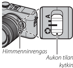
Himmenninrenkas
