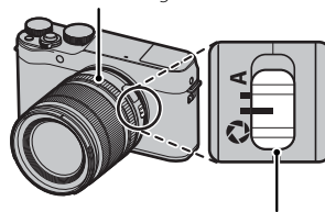
Bländarlägesväljare
